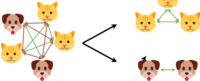
Рис. 1: Иллюстрация задачи двустороннего разбиения
