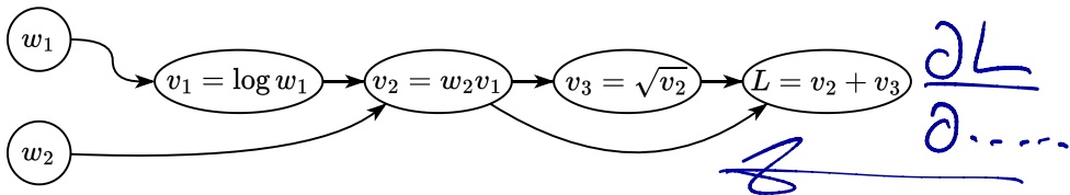
Рис. 20: Иллюстрация вычислительного графа для функции L(w_1, w_2)
