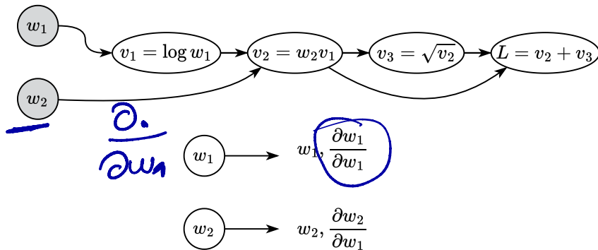
Рис. 9: Иллюстрация прямого режима автоматического дифференцирования
